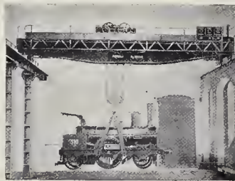
Gru elettrica a ponte costruita dalle Officine di Savigliano.
